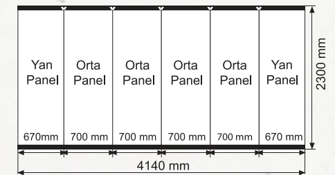
3x4 Oval Baskı Alanı
